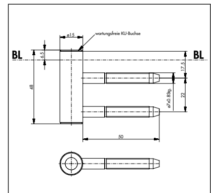
Rahmenteil für Holzzargen wartungsfrei, 50 mm
